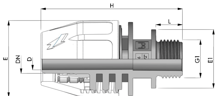
Rechte koppeling
