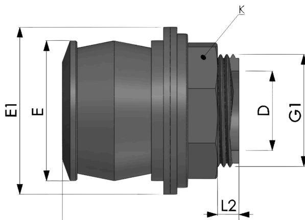
Tankadapter huiddoorvoer
